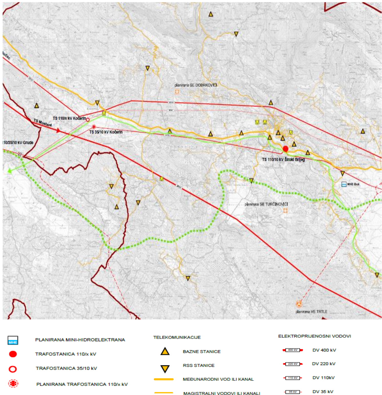
Slika 5. Elektroenergetske građevine za proizvodnju i prijenos električne energije
