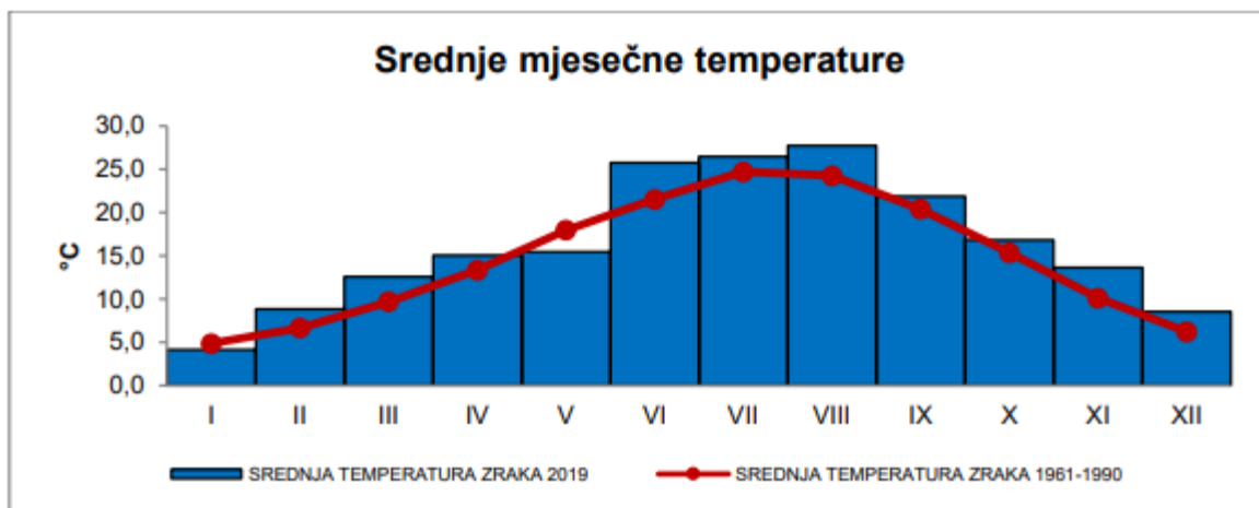
Grafikon 2. Srednje mjesečne temperature (°C)
